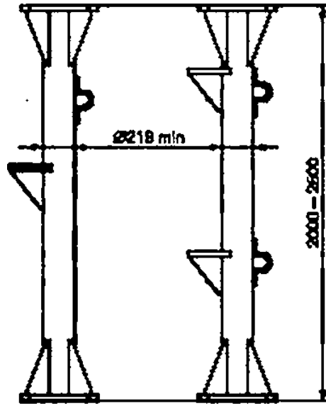
Рисунок 2 — Схема вертикальных опор
